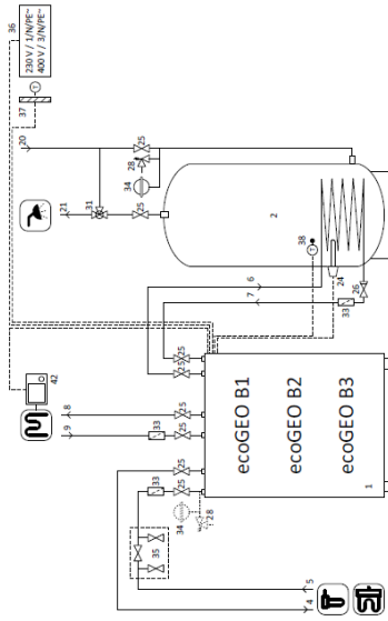
Figuur 14.1. Installatieschema monozone voor ecoGEO B1, B2 en B3.
